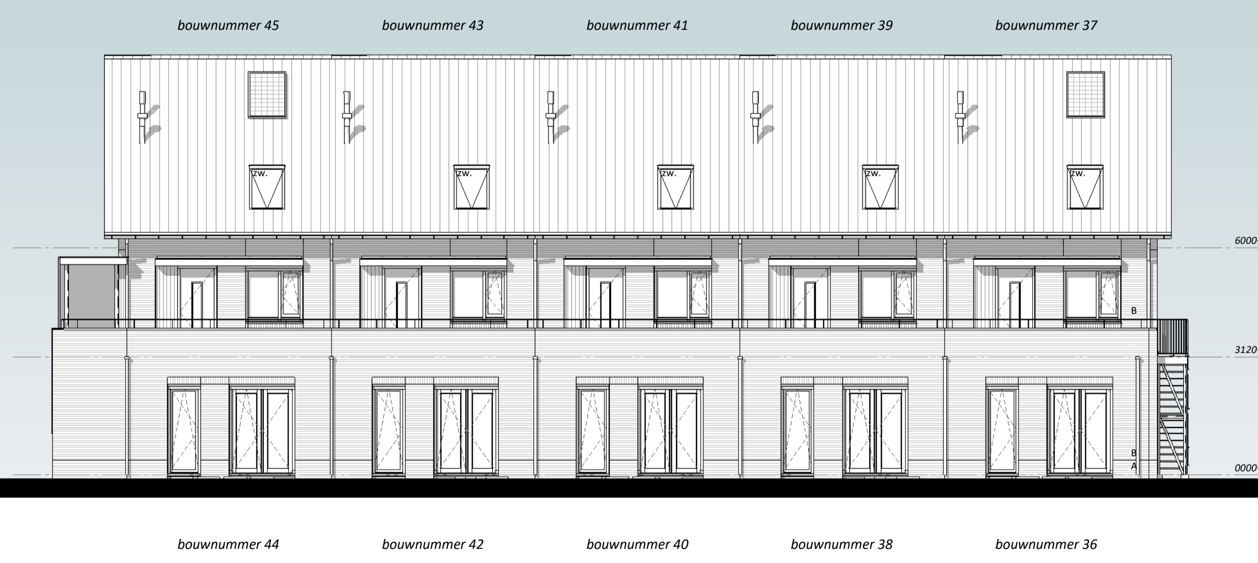
achtergevel
