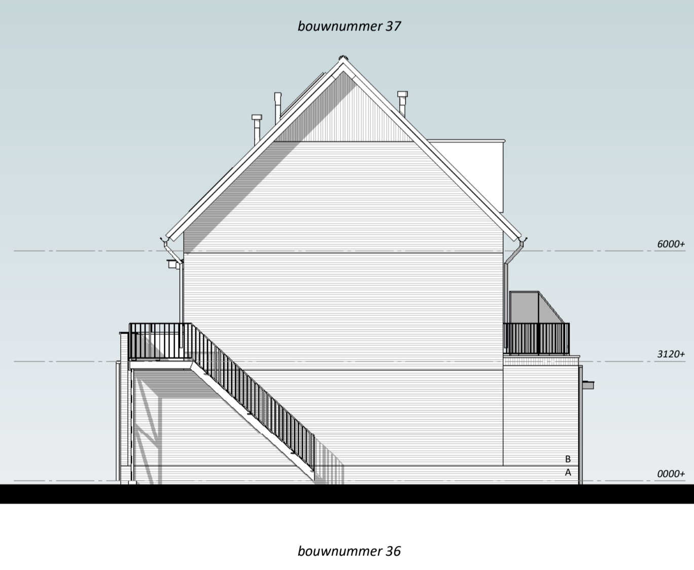
linkergevel
