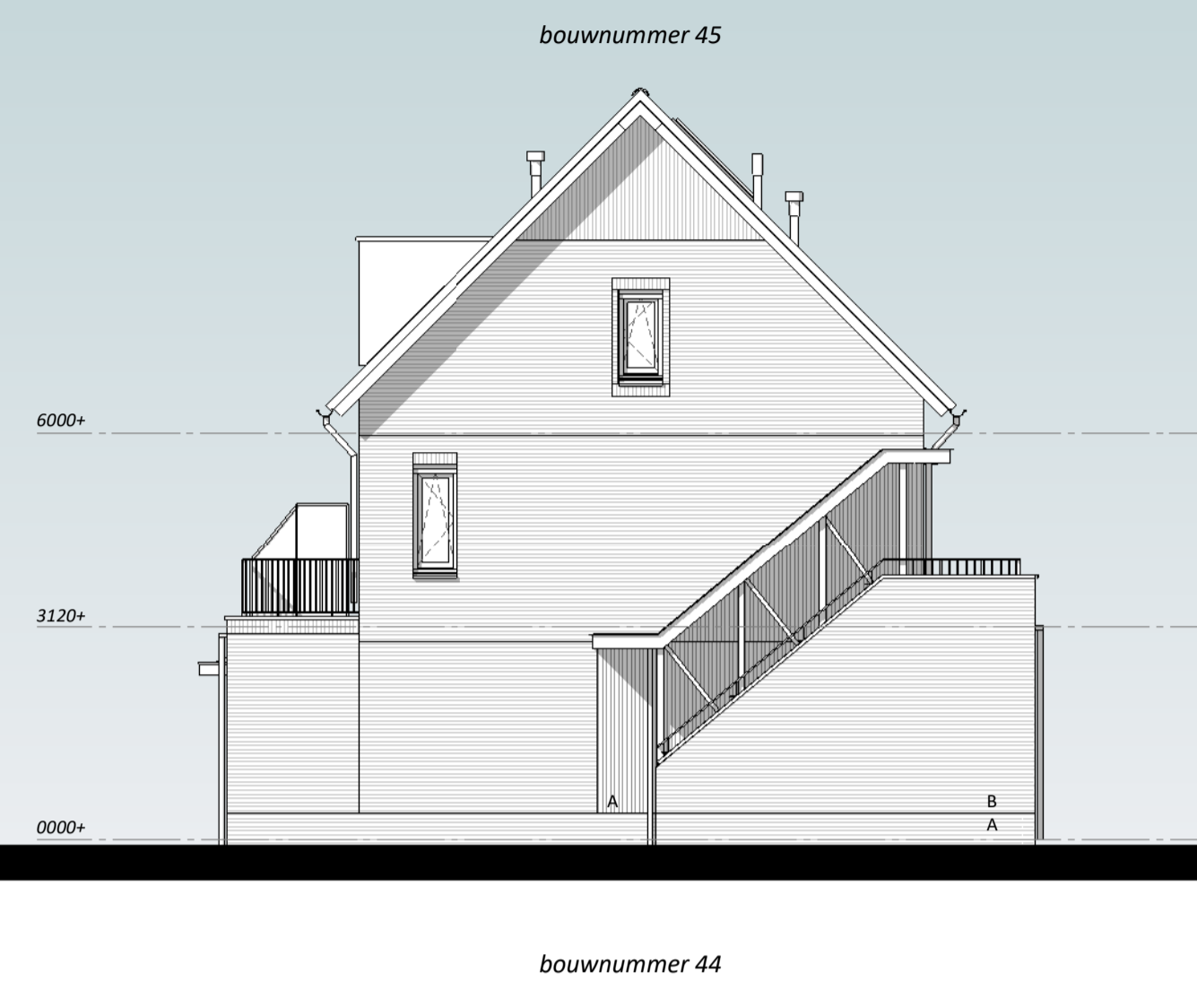
rechtergevel
