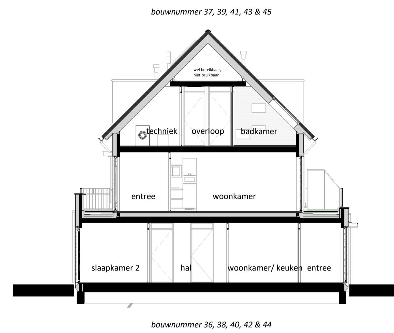
doorsnede
